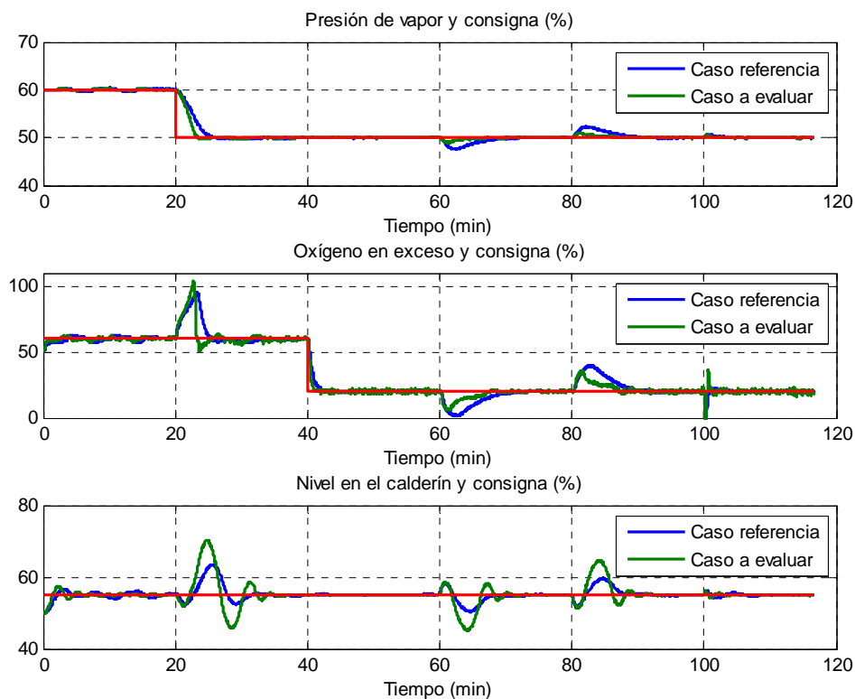
Figura 6b Respuestas del proceso, Puntos de consigna (rojo) y variables controladas. Los trazos en azul corresponden al primer ajuste de los controladores PID (elegido como el Caso referencia) y los trazos en verde corresponden al segundo ajuste (corresponde al Caso que se quiere evaluar).
