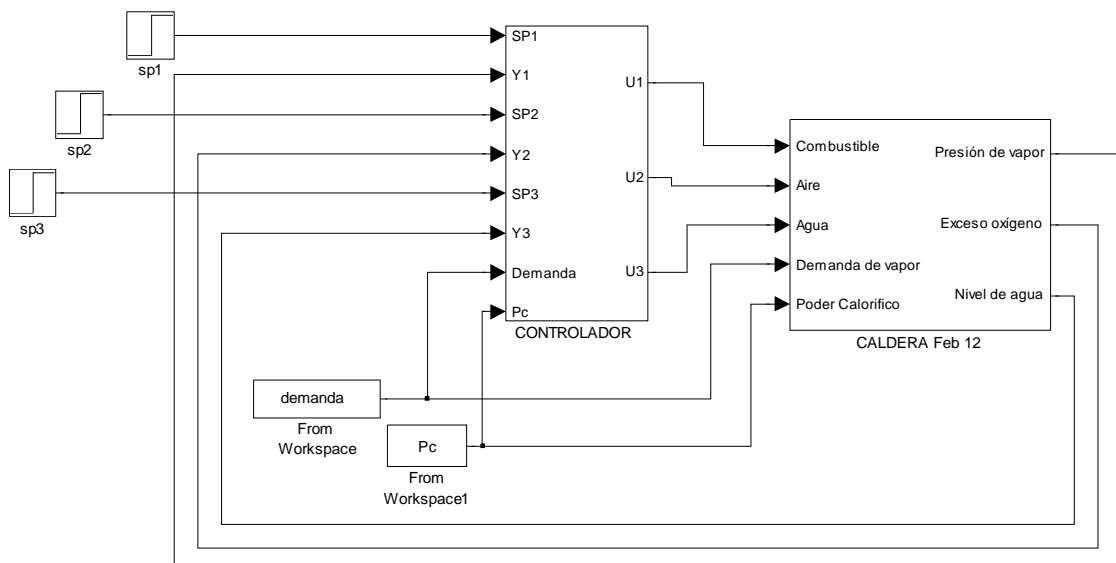
Figura 3 Esquema Simulink del sistema de control de la caldera.
