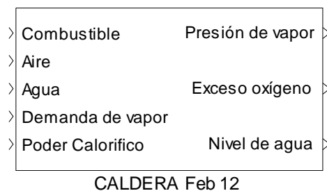
Figura 2 Bloque MIMO que representa a la caldera
