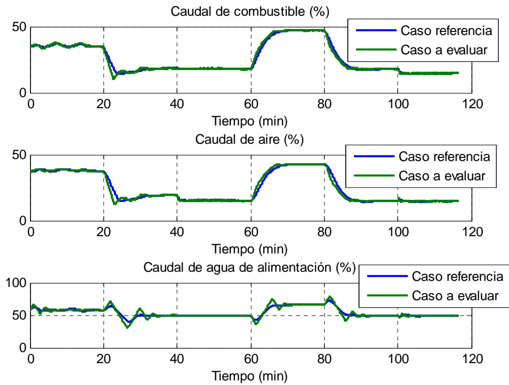
Figura 6c Respuestas del proceso, Variables manipuladas. Los trazos en azul corresponden al primer ajuste de los controladores PID (elegido como el Caso referencia) y los trazos en verde corresponden al segundo ajuste (corresponde al Caso que se quiere evaluar).
