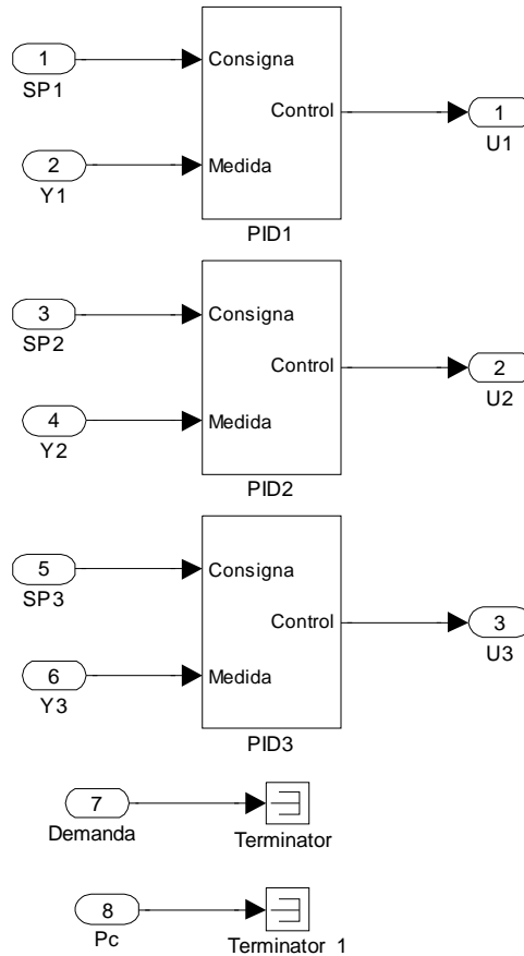
Figura 4 Esquema Simulink del controlador descentralizado
