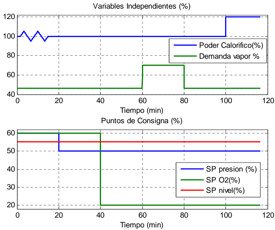
Figura 6a: Patrón de movimientos en las variables independientes.
