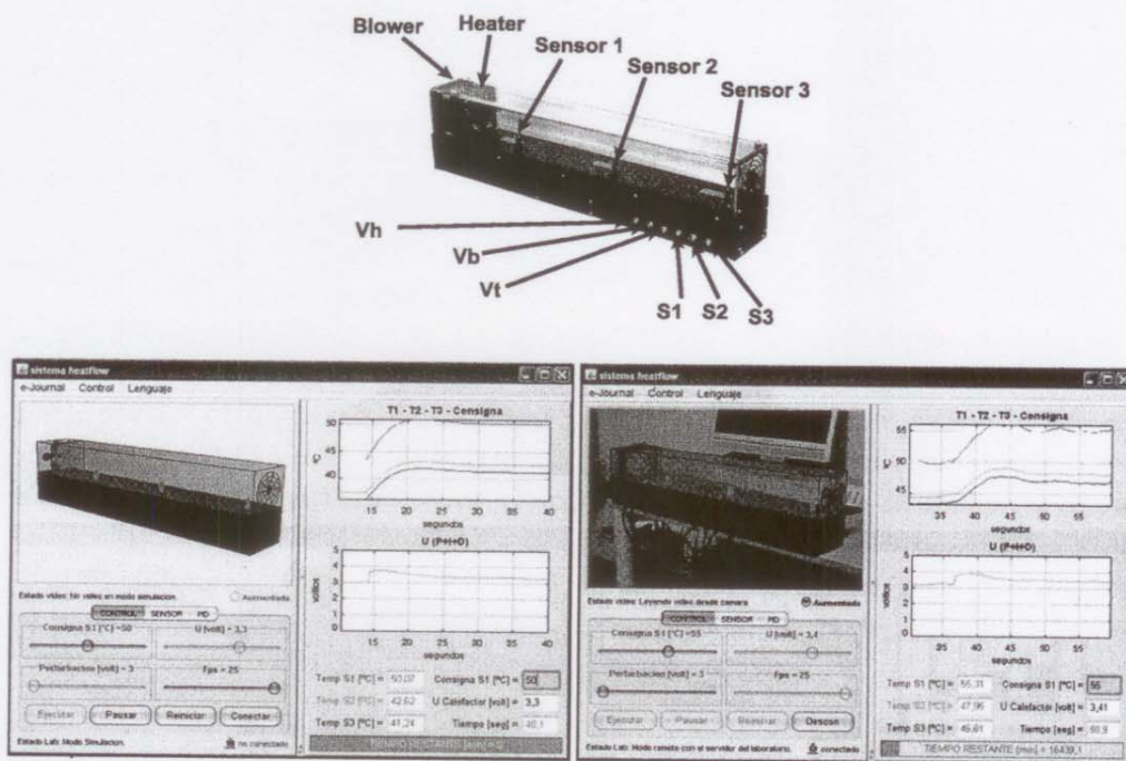
Figura 4. El sistema heatflow.
