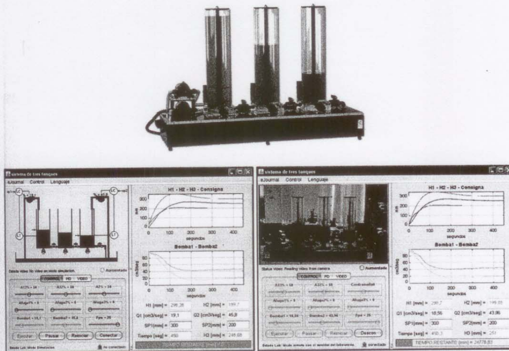
Figura 3. El sistema de tres tanques.
