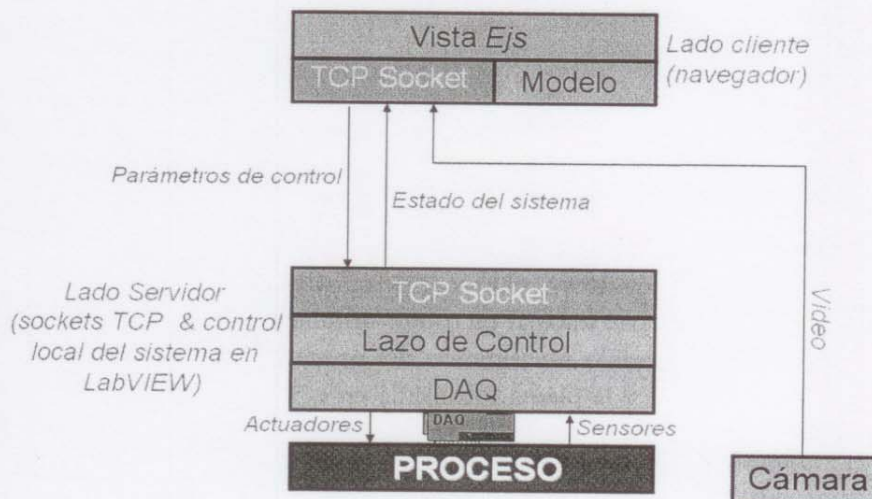
Figura 2. Estructura de comunicación Ejs/LabVIEW.
