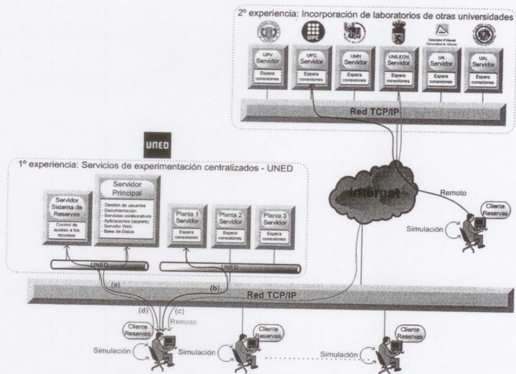
Figura 1. Infraestructura de red y servicios web.
